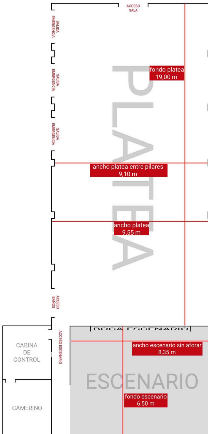
Imagen 5: Croquis de la sala
