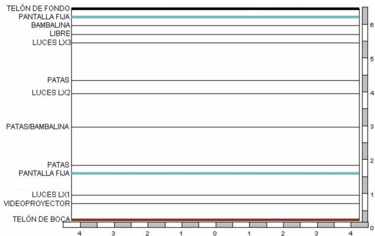
Imagen 6: Plano de varas y plano de luces
